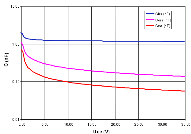
Typ. capacitances
