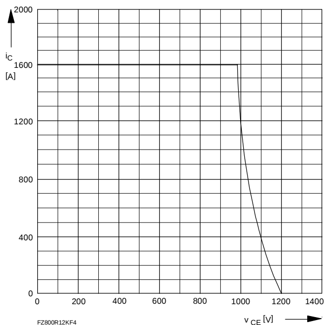
Bild/Fig. 4 Rückwärts-Arbeitsbereich Reverse biased safe operating area t_{vj} = 125\text{ °C} , v_{LE} = v_{LR} = 15\text{ V} , R_G = 1,8\text{ W}
