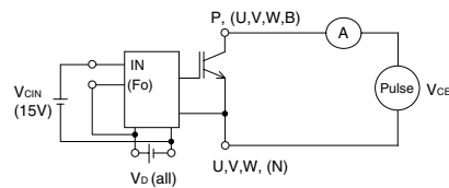
Fig. 4 I_{CES} Test
