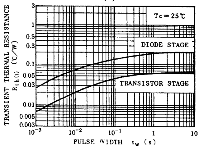
R_{th}(t) - t_w
