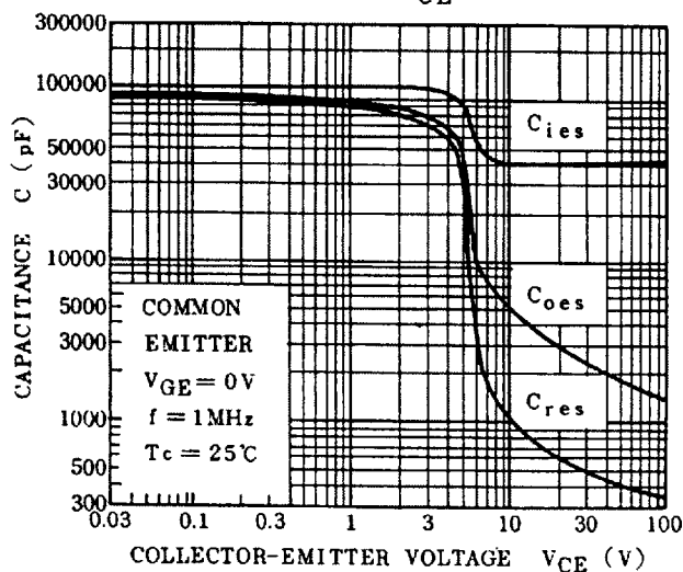
C - V_{CE}
