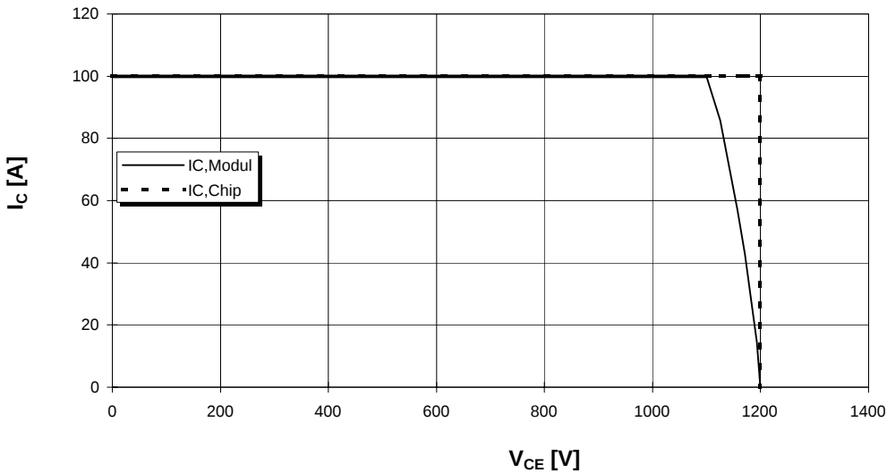
Sicherer Arbeitsbereich (RBSOA) Reverse bias safe operation area (RBSOA) V_{GE} = 15V, R_g = 15 \text{ Ohm}, T_{vj} = 125^\circ C
