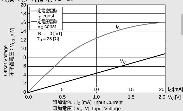
V_{OS}-V_C, V_{OS}-I_C (参考)
