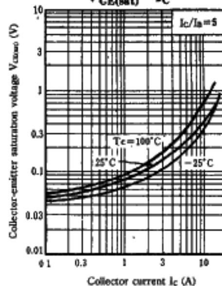
V_{CE(sat)} - I_C
