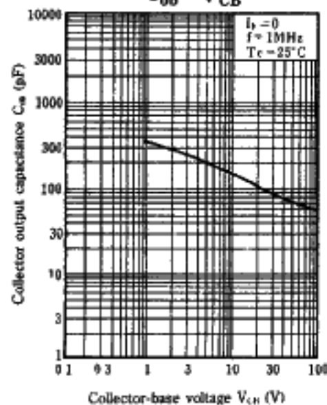
C_{ob} - V_{CB}
