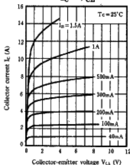
I_C - V_{CE}
