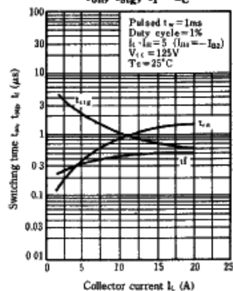
t_{on}, t_{stg}, t_f - I_C
