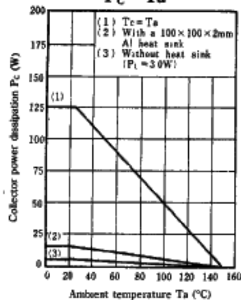
P_C - T_a
