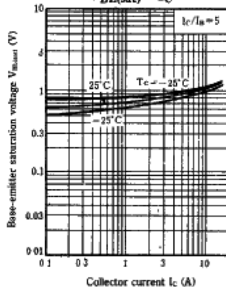
V_{BE(sat)} - I_C
