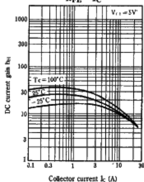
h_{FE} - I_C
