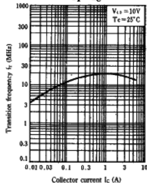
f_T - I_C
