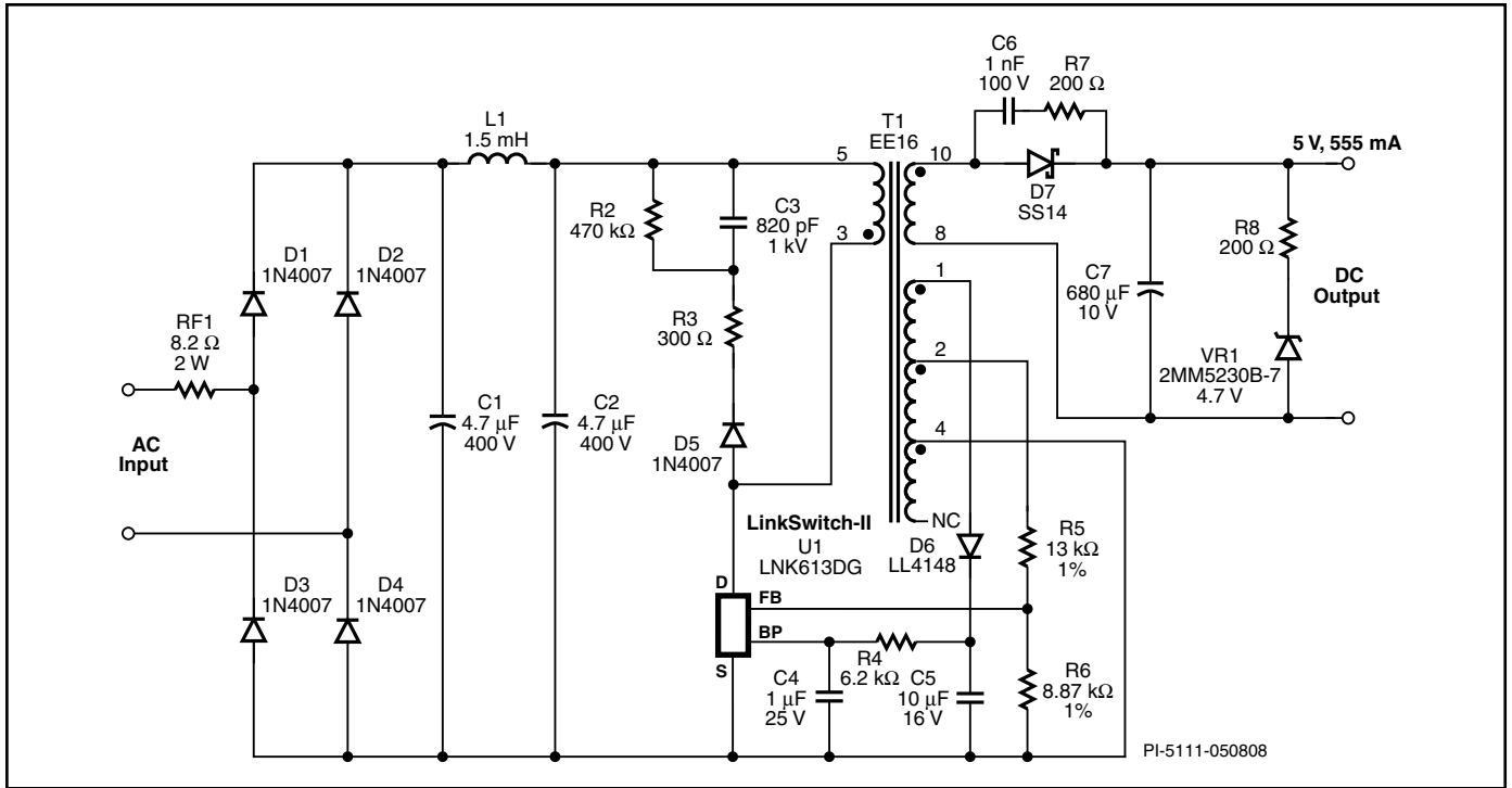
图4. 高效USB充电器电源（平均效率为74%，空载输入功率&lt;40 mW）
