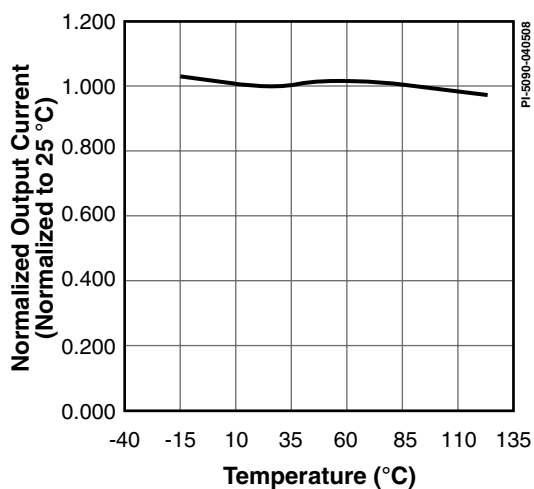
图 14. 归一化输出电流与温度的特性曲线
