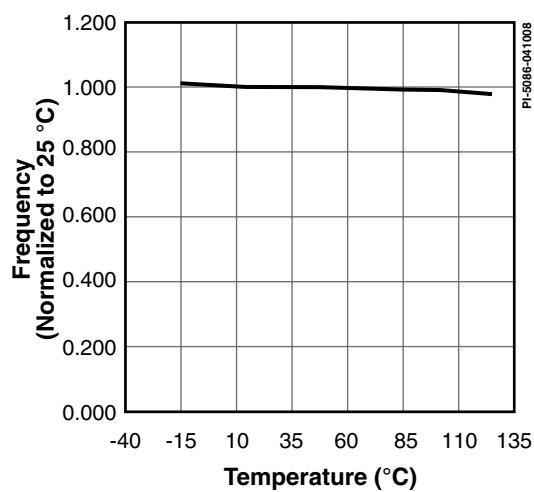
图 10. 输出频率与温度的特性曲线
