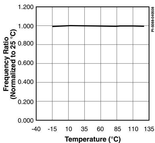
图 12. 频率比与温度（电感电流）的特性曲线
